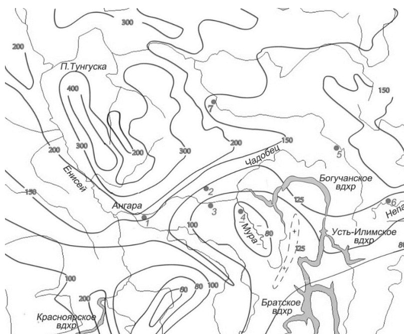
Рисунок 2 – Средние многолетние запасы воды в снеге (мм) перед началом снеготаяния
