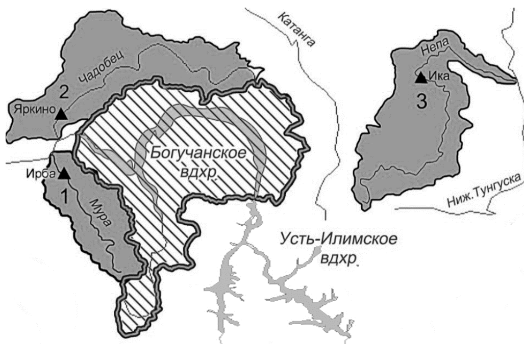
Рисунок 3 – Схема расположения рек – аналогов Примечание – бассейны рек: 1 – Мура; 2 – Чадобец; 3 – Непа. Штриховкой выделен бассейн Богучанского водохранилища
