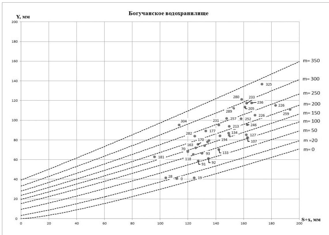
Рисунок 4 – Зависимость Y = f(S + X, m)
