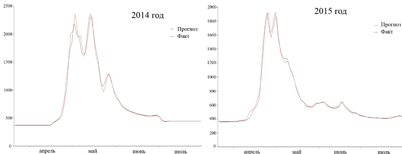
Рисунок 6 – Гидрограф бокового притока в Богучанское водохранилище
